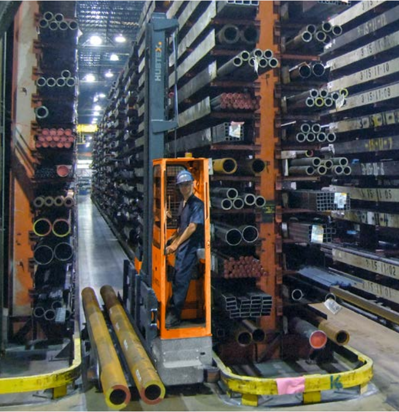
Dar koridorda çok yönlü yanal istifleyici Multidirectional-Sideloader in narrow aisle application
