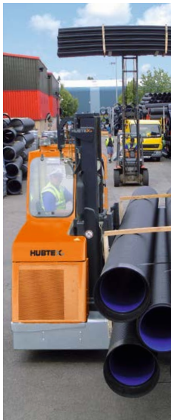
Dizel veya LPG tahrikli, üniversal dört yönlü yanar istifleyici Diesel- or LPG-powered Fourway-Sideloader
