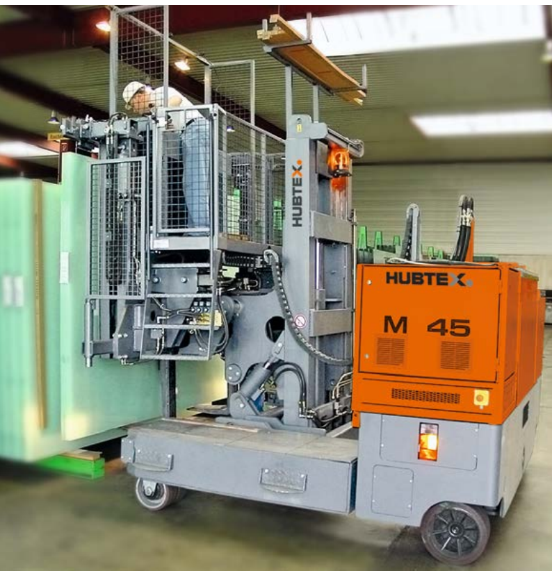
Mehrwege-Seitenstapler für das Handling von unverpackten Glaspaketen Multidirectional-Sideloader for handling of unpacked glass packs
