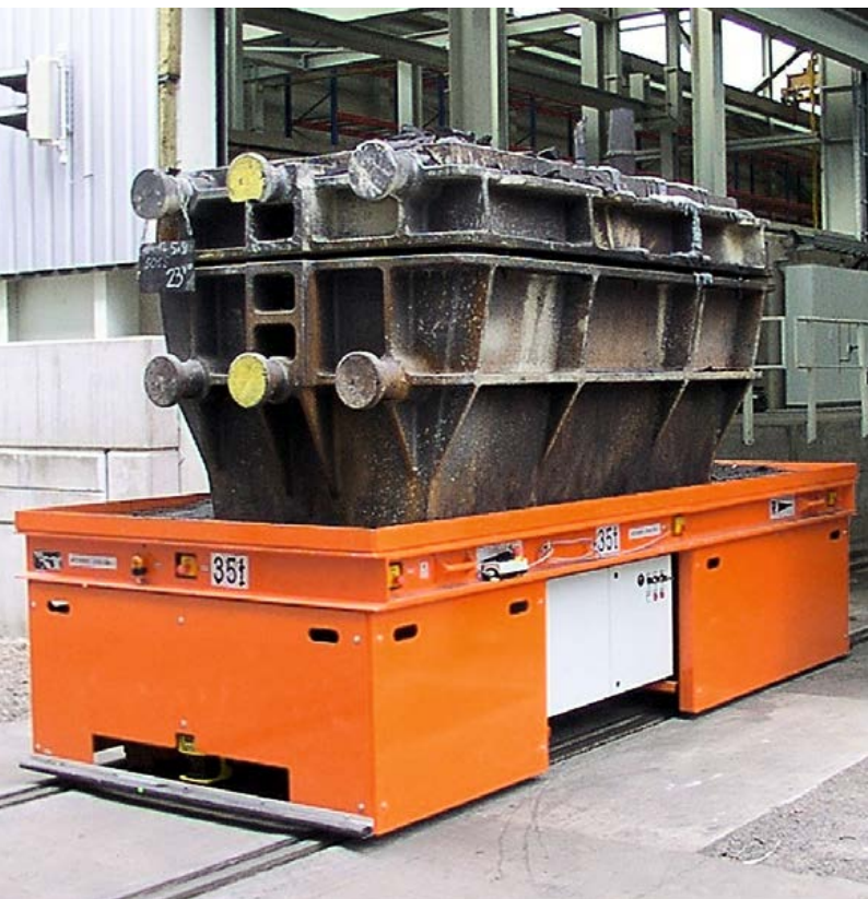
Gleiswagen zum Transport von Gussformen Rail car for mould transport
